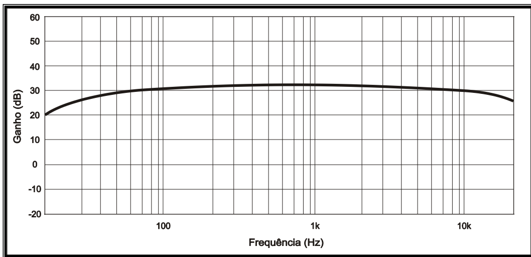
Figura 1 – Resposta em Frequência da Magnitude.
