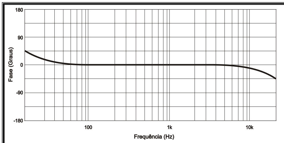
Figura 2 – Resposta em Frequência da Fase.
